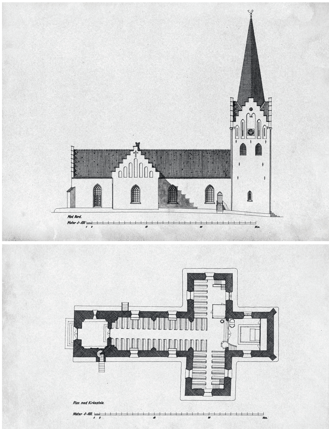
Fig. 27a-b. Opmåling af kirken. Målt og tegnet af Jørgen Ejlers 1940. 1:400. a. Nordfacader. b. Plan med stoleinddeling. I Svanninge Folkemindesamling. — Scale drawing of the church, 1940. a. North facades. b. Plan with pew layout.
