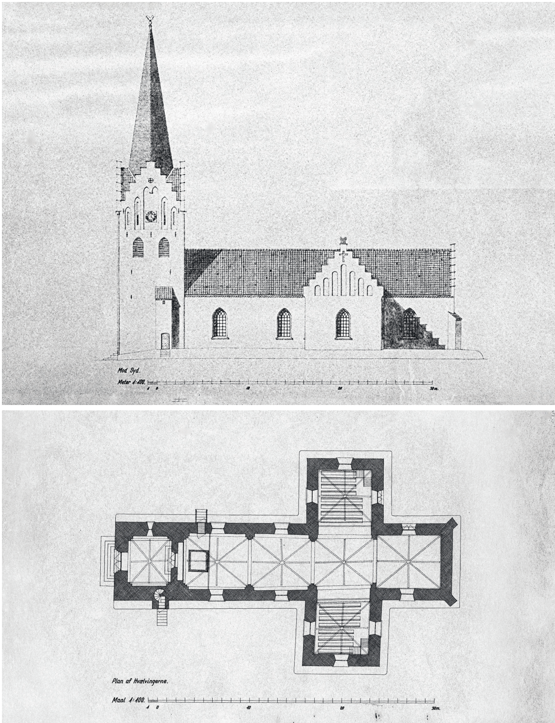
Fig. 27c-d. Opmåling af kirken. Målt og tegnet af Jørgen Ejlers 1940. 1:400. c. Sydfacader. d. Plan af pulpiturer og hvælv. I Svanninge Folkemindesamling. — Scale drawing of the church, 1940. c. South facades. d. Plan of galleries and vaults.
