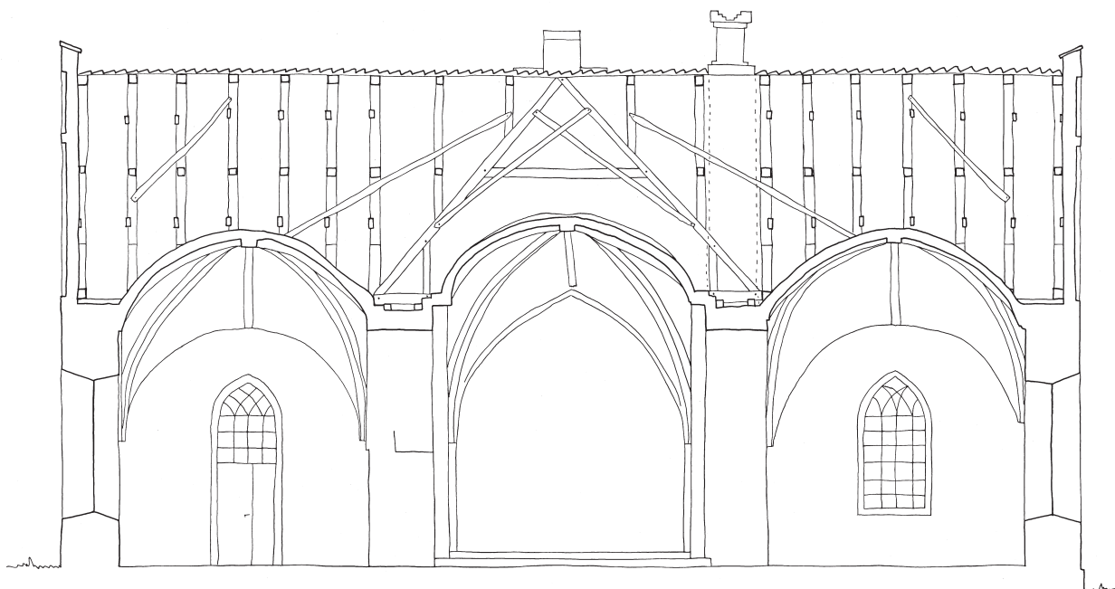
Fig. 13. Tværsnit. 1:150. Målt og tegnet af Pia K. Lindholt 2025. – Cross-section.
