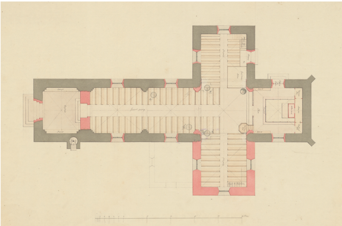
Fig. 21a. Forslag til hovedistandsættelse tegnet af G. F. Hetsch 1836. 1:300. a. Grundplan. I KB. Kunstbiblioteket. – Proposal for major refurbishing by G. F. Hetsch, 1836. a. Plan.
