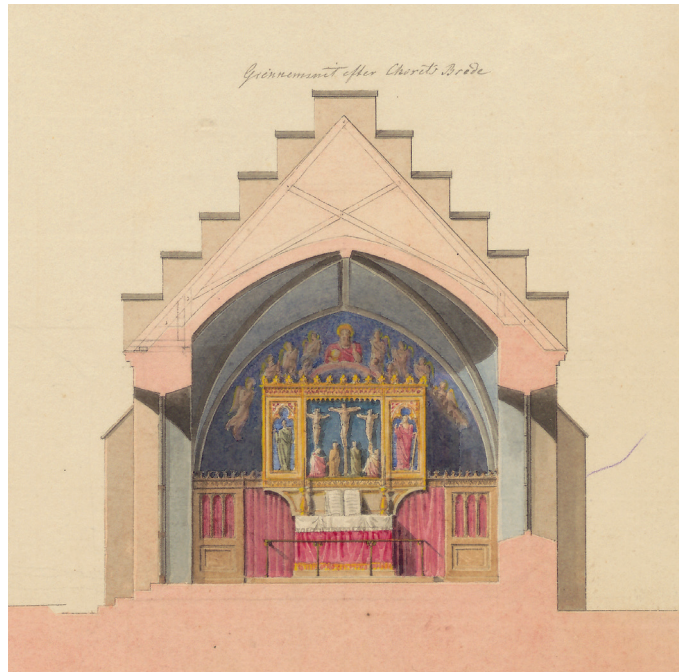
Fig. 21f. Forslag til hoveddistandsættelse. Tegnet af G. F. Hetsch 1836. 1:150. f. Tværsnit gennem koret set mod øst. I KB. Kunstbiblioteket. – Proposal for major refurbishing by G. F. Hetsch, 1836. f. Cross-section through the chancel looking east.
